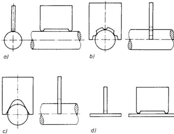
figuur 3.7 Voorbeelden van gestante langwerpige projecties
