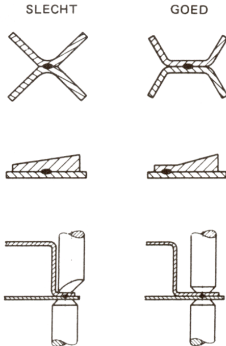
figuur 8.11 Voorbeelden van constructievormen met goede en slechte aanligvlakken
