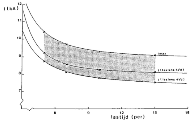
figuur 2.10 Lasstroomsterkte in afhankelijkheid van lastijd voor éénzijdig verzinkt IF staal met d = 0,7 \text{ mm}
