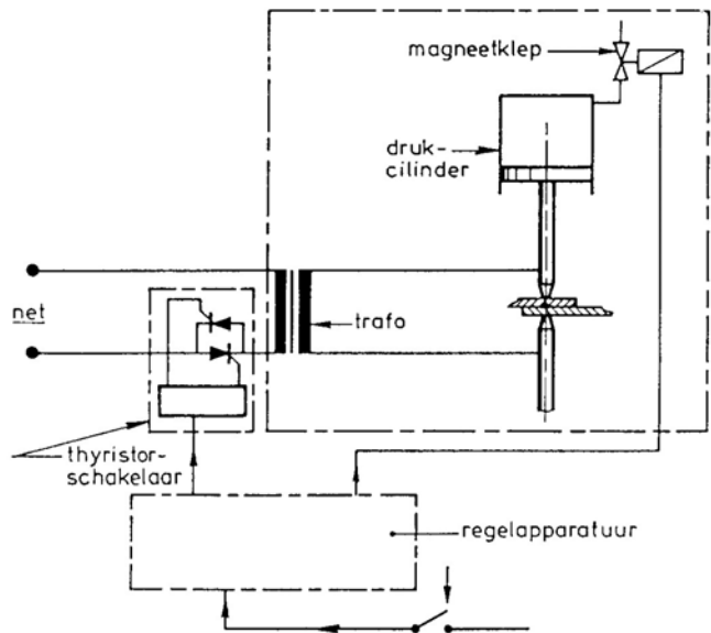
figuur 4.5 Schematische voorstelling van een weerstandslasmachine met regel- en schakelapparatuur
