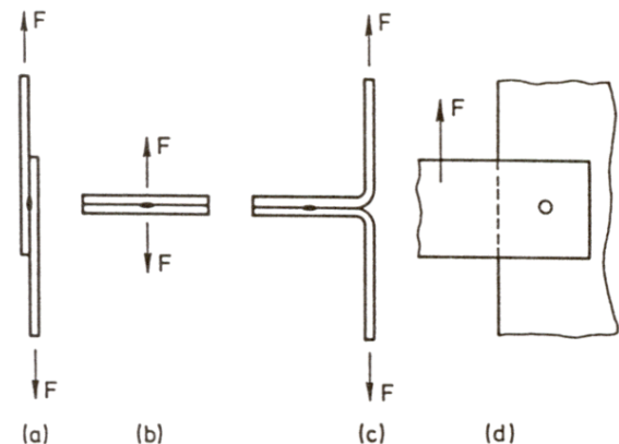
figuur 8.2 Belastingvormen voor een puntlasverbinding
