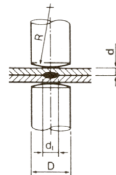
figuur 10.5 Grootheden bij het puntlassen (zie tabel 10.5)
