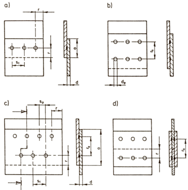
figuur 8.1 Voorbeelden van puntlaspatronen en definitie van bijbehorende geometrische grootheden
