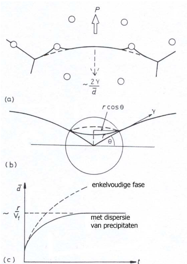
Figuur 2 - Schematische voorstelling van het pinnen van korrelgrenzen door precipitaten (a), de invloed van een precipitaat op de totale oppervlakte-energie (b), het verschil in gemiddelde korrelgrootte voor een enkelvoudige fase en een metaal met een dispersie van precipitaten als functie van tijd (c) [6]
