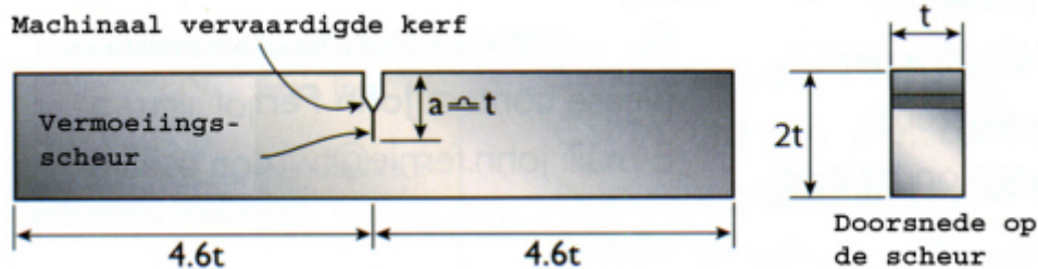
Figuur 1 - Buigproefstuk voor CTOD-metingen met een proportionele rechthoekige doorsnede.
