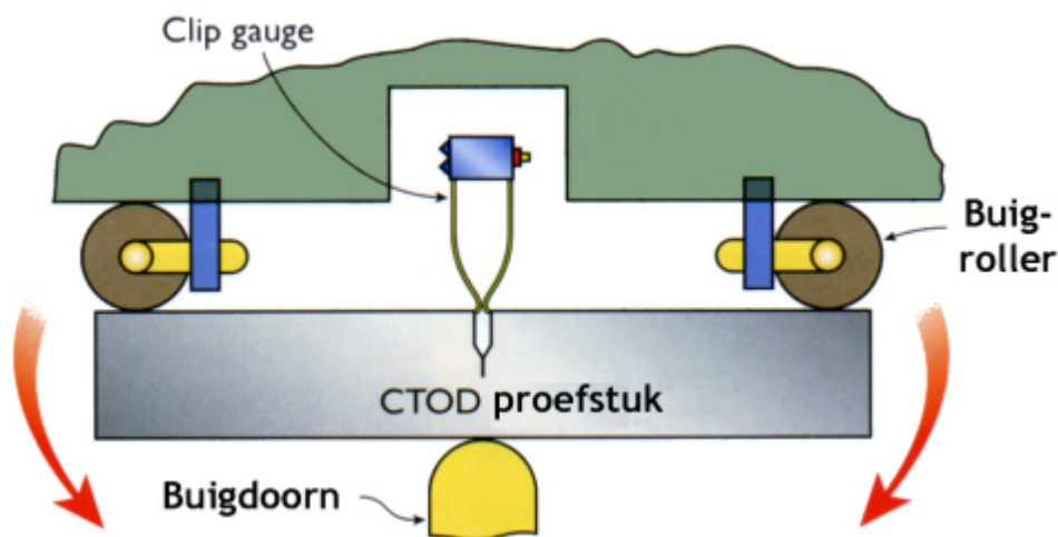
Figuur 2 - Kenmerkende proefopstelling. Het proefstuk kan gemakkelijk ondergedompeld worden in een bad met een lage temperatuur.
