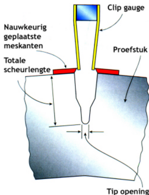
Figuur 3 - Positie van het CTOD-proefstuk, onmiddellijk voorafgaande aan scheuruitbreiding.
