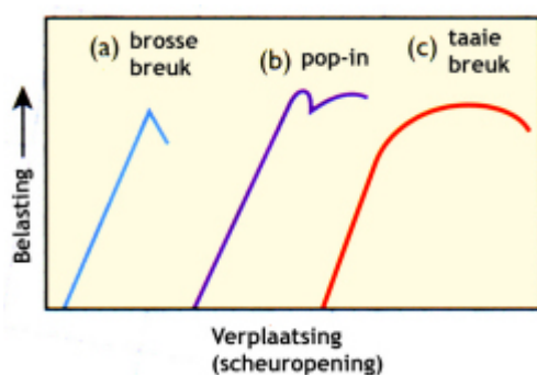
Figuur 4 - De belasting uitgedrukt tegen de scheuropeningsverplaatsing. Drie kenmerkende typen van scheurgedrag.
